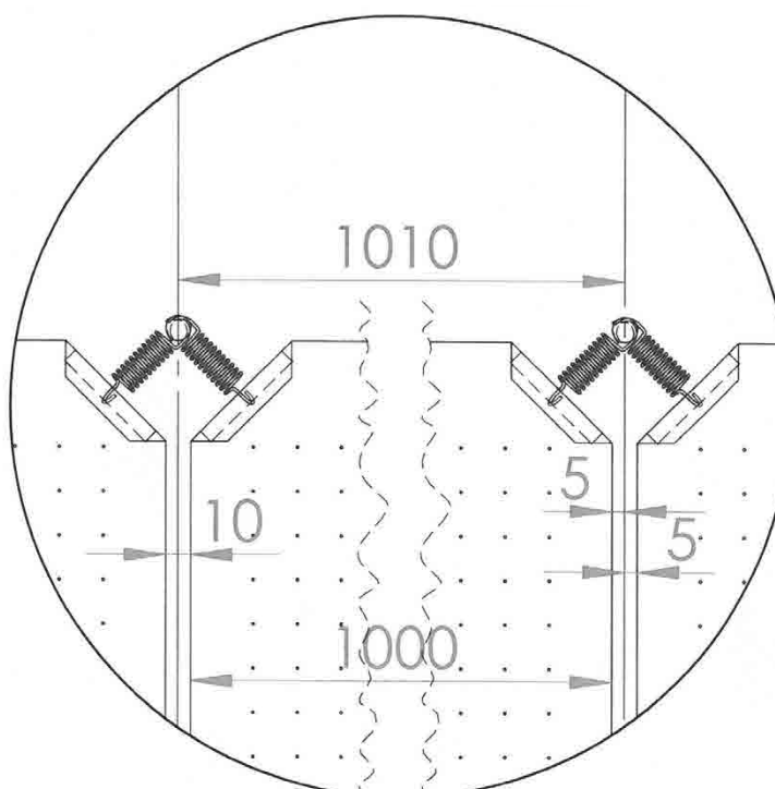
Détail pour une toile Microsorber® pour piscines
