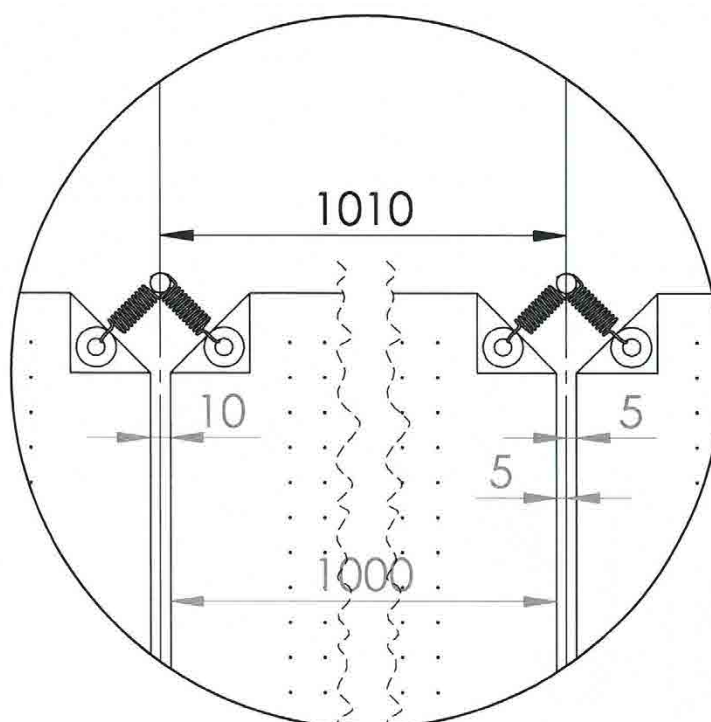
Détail pour une toile Microsorber® classique
